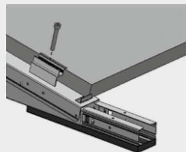
Solarmodul (bereitgestellt vom Installateur)
