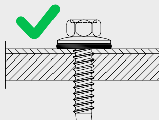
Serraggio corretto
